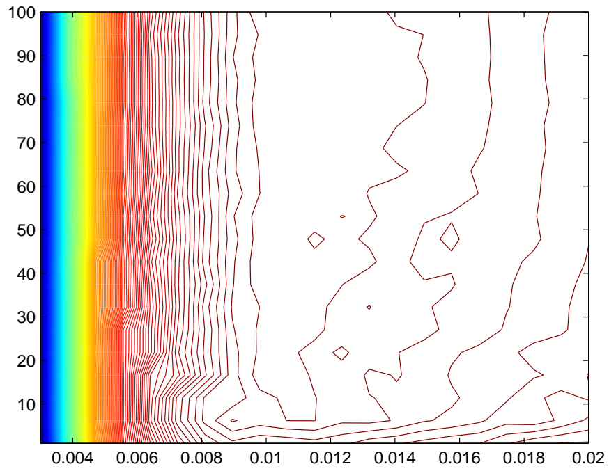
(a) Posterior
